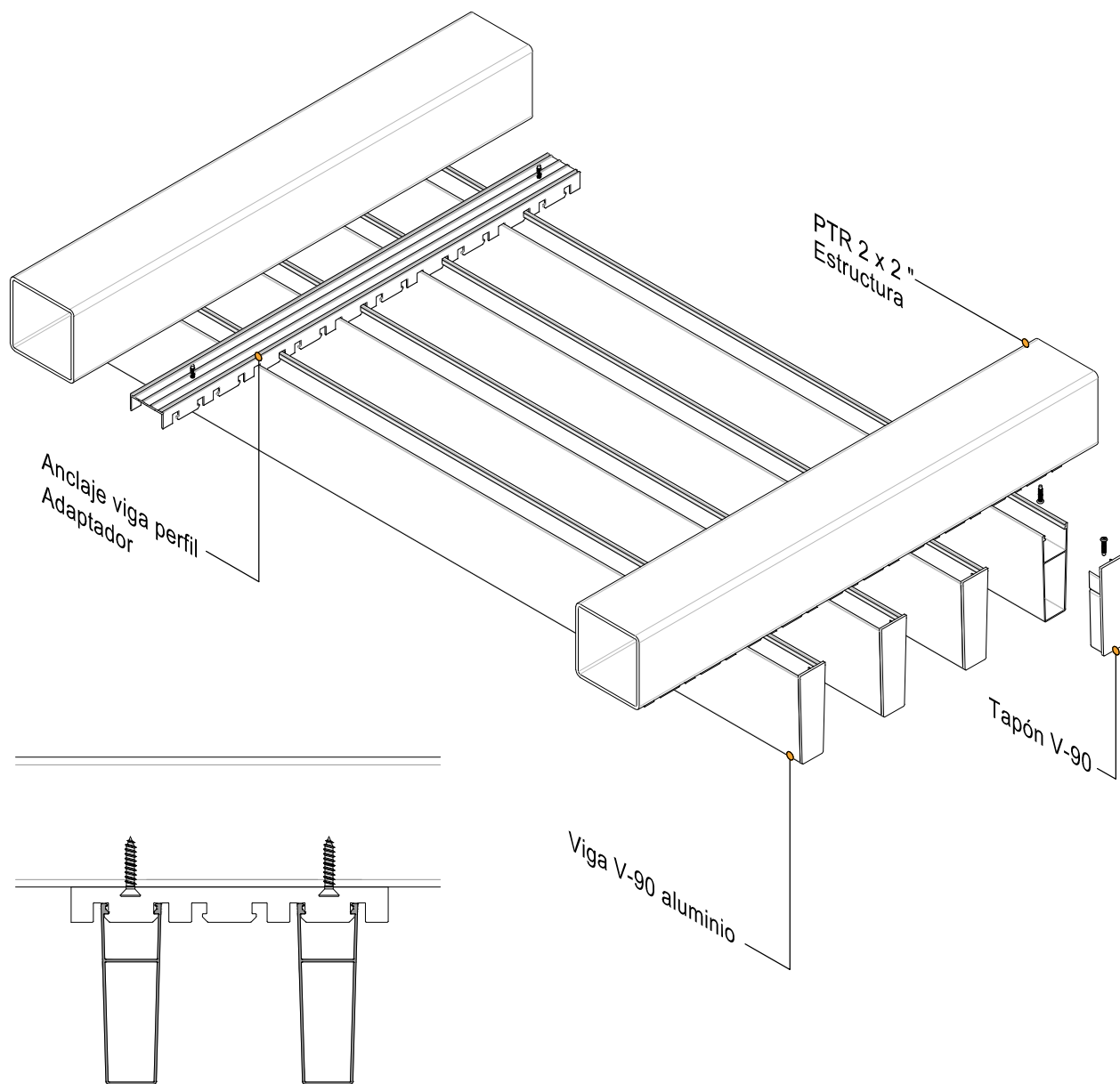
DETALLE ANCLAJE VIGA V-90 A ESTRUCTURA DE ACERO
